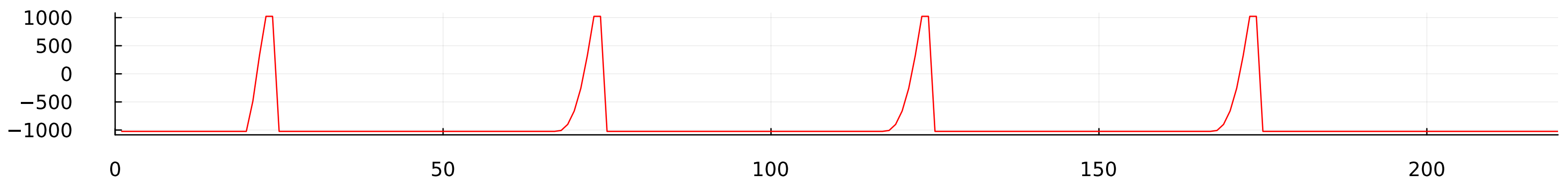
h(Z_{hyp}=1000)
