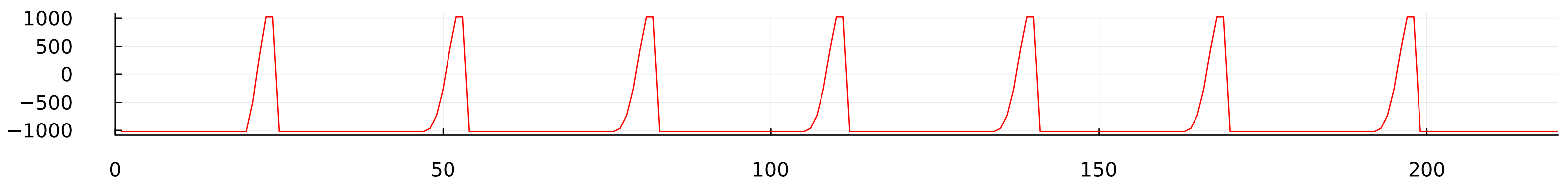
h(Z_{hyp}=960)
