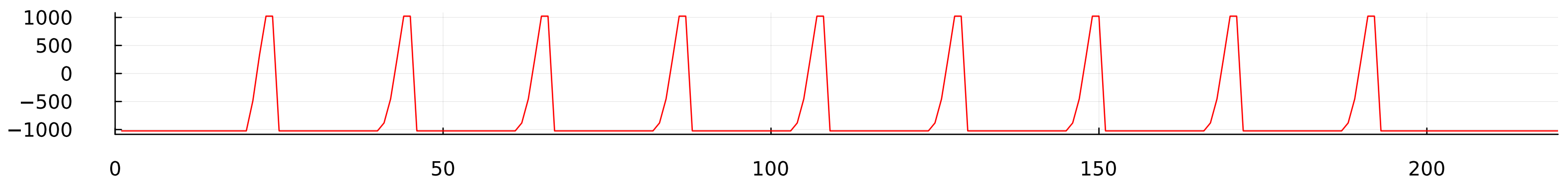
h(Z_{hyp}=920)
