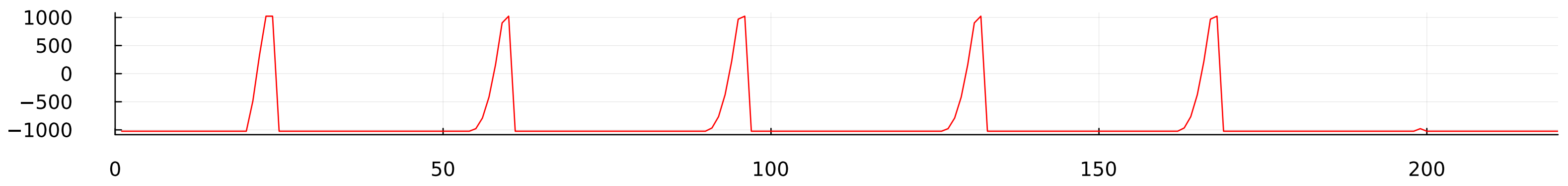
h(Z_{hyp}=980)
