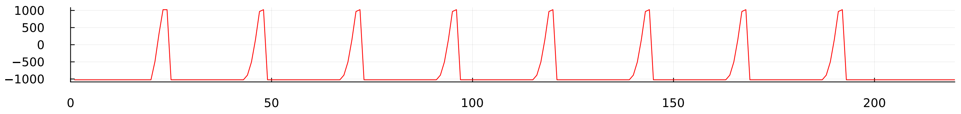
h(Z_{hyp}=940)
